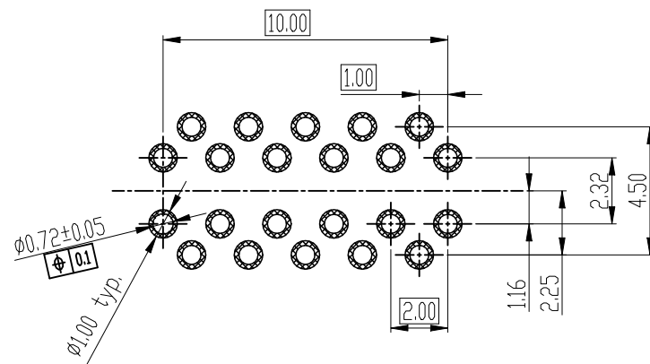
Recommendde P.C.B Layout(±0.05)
